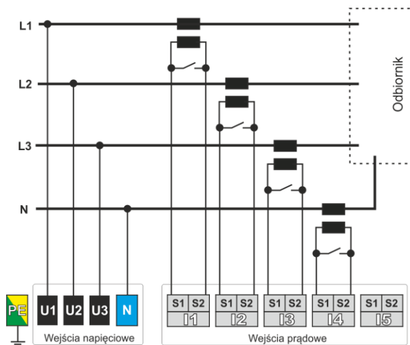
Rys. 27. Schemat podłączenia – układ 3-fazowy 4-przewodowy, bezpośrednie podłączenie napięć.
