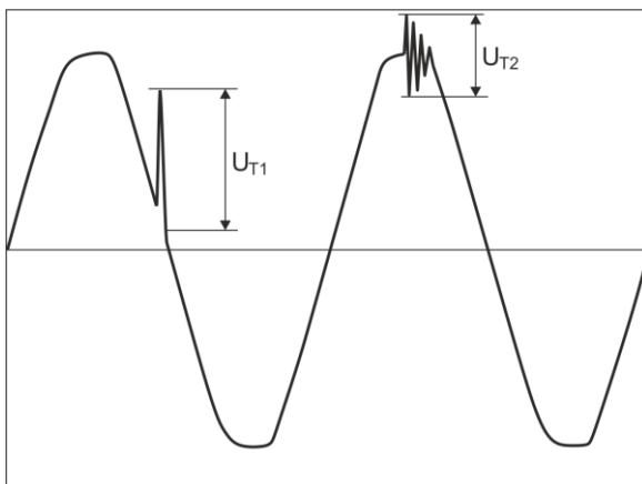
Rys. 36. Sposób wyznaczania amplitud transjentów.
